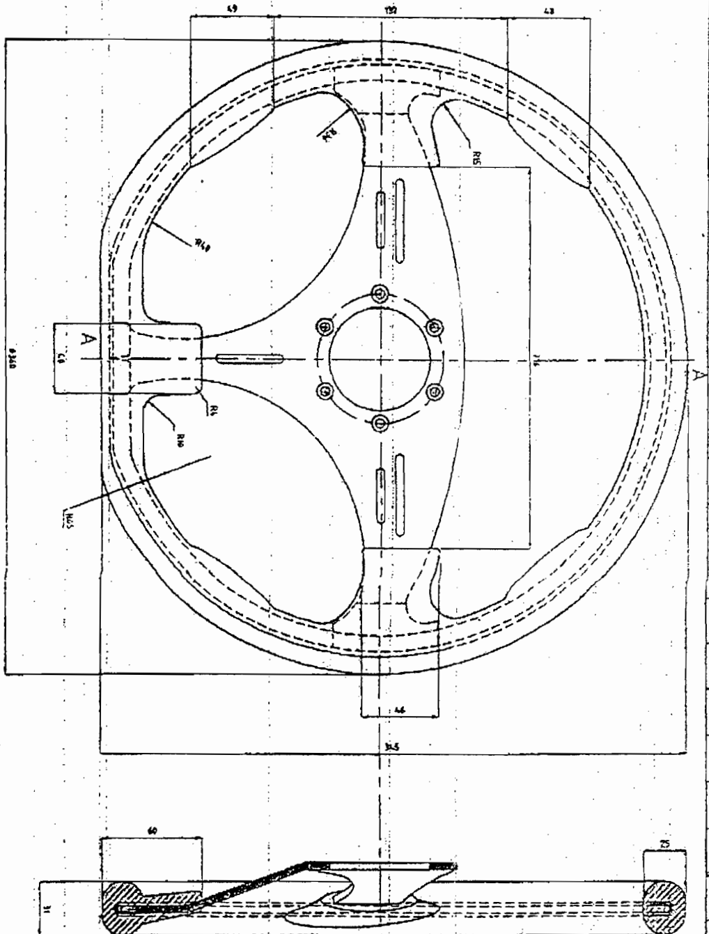
SEZIONE A-A
